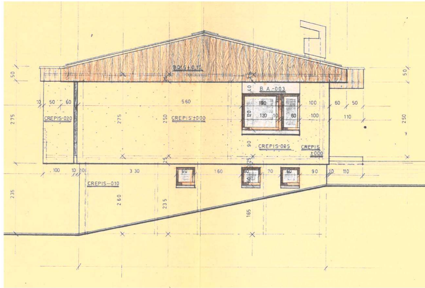
Coupe de la façade
